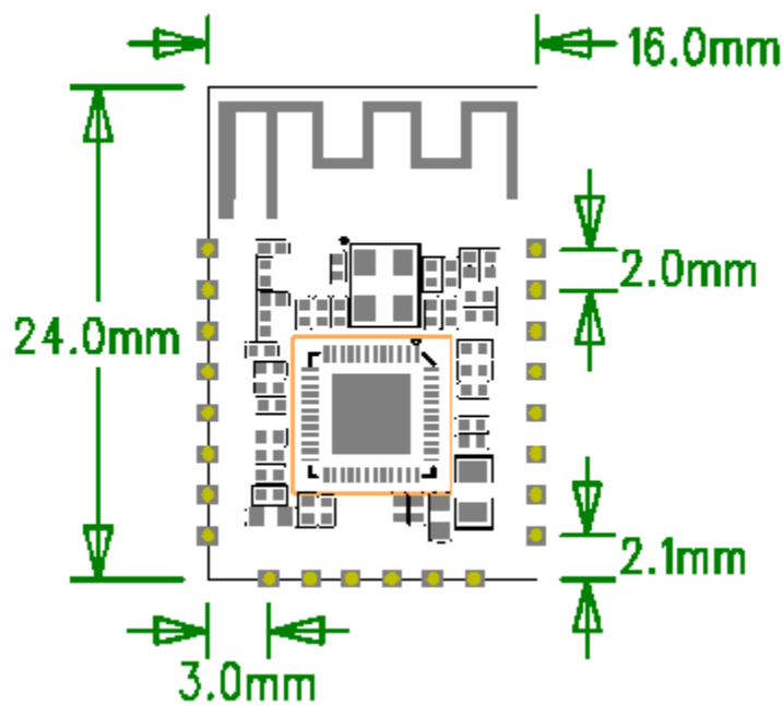
图 4 RTL00 模组尺寸平面面图
