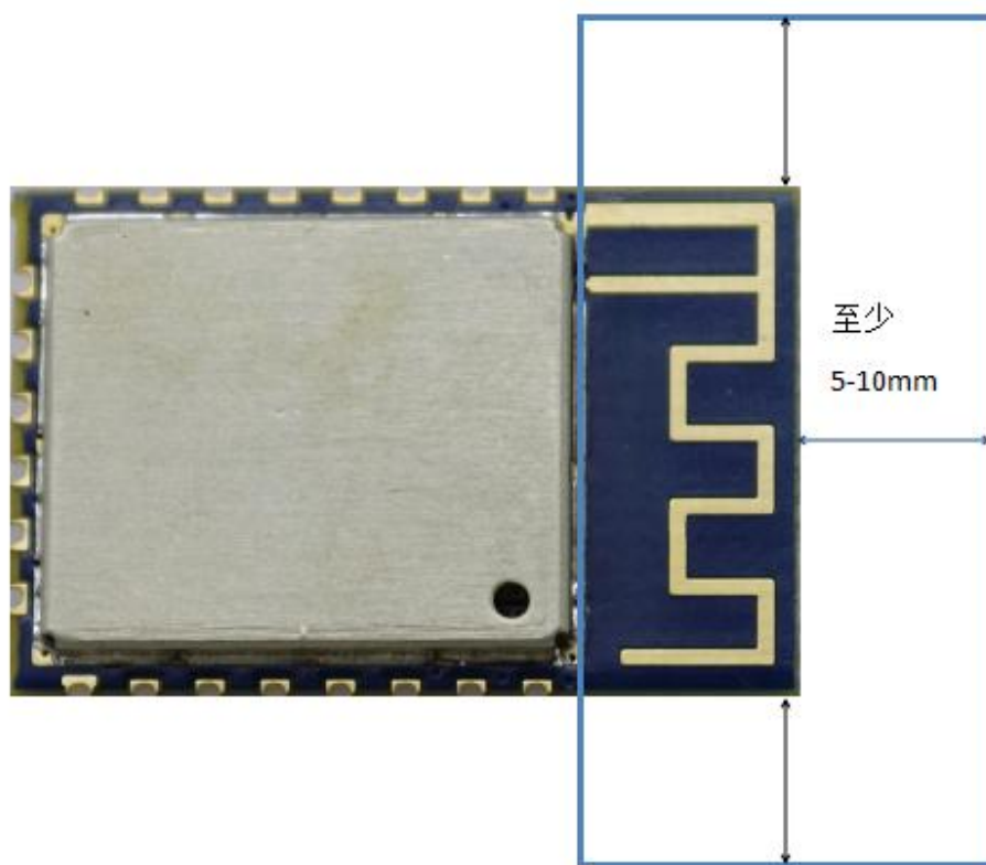
正面图 图 5
