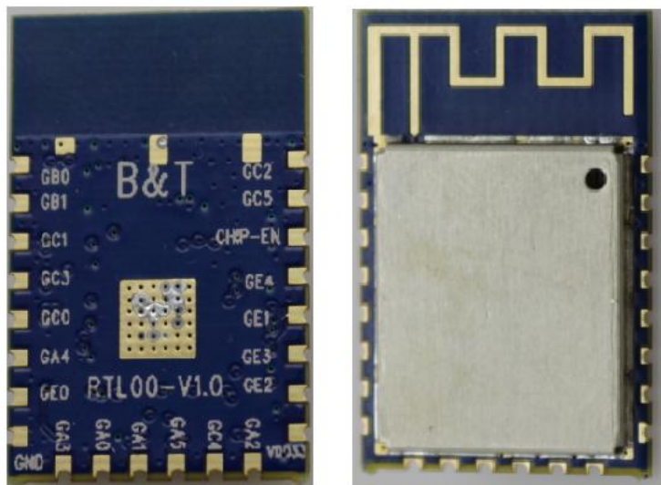
图 3 RTL00 模组外观
